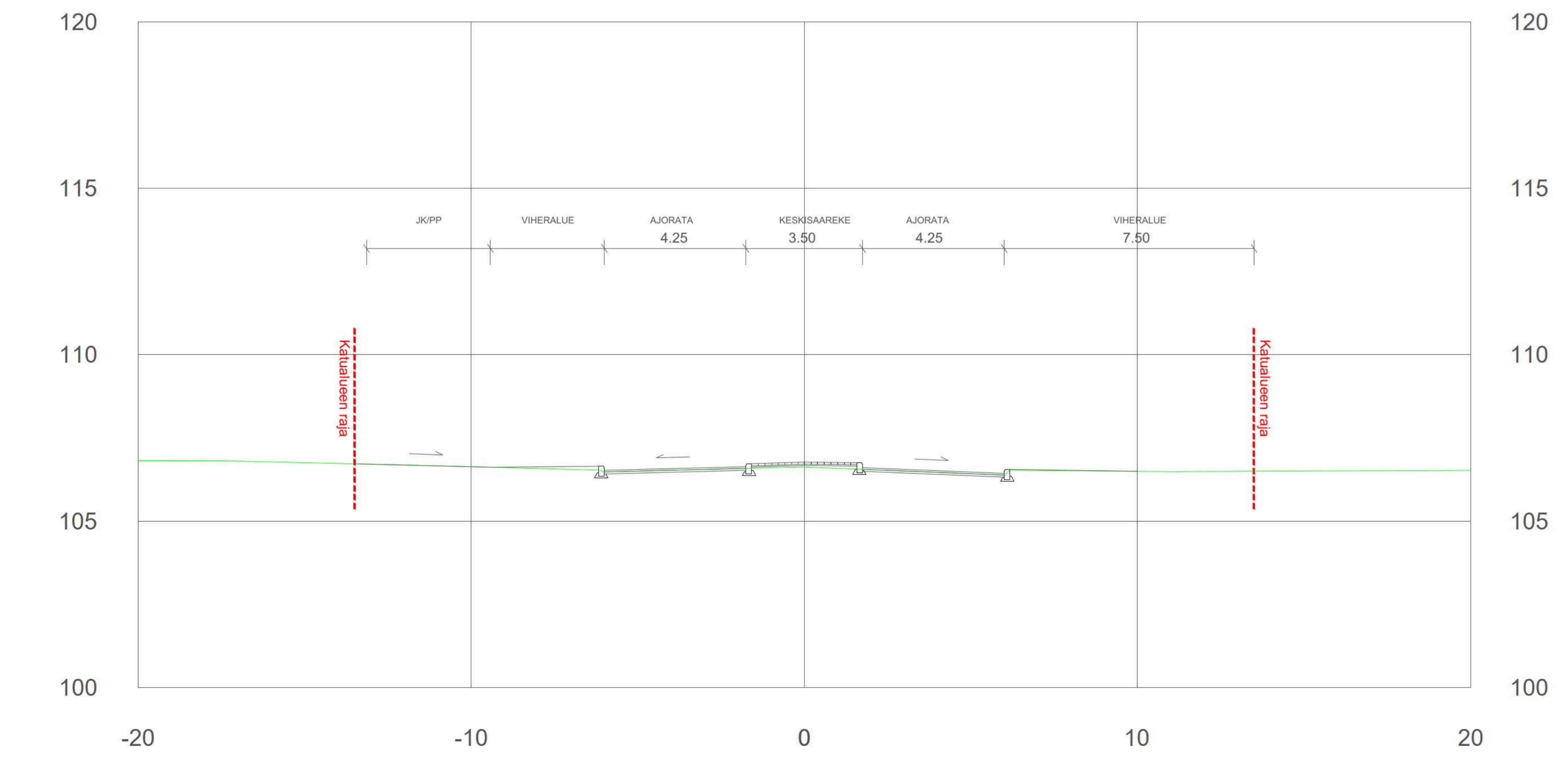
A-A PL120 / 1:100
