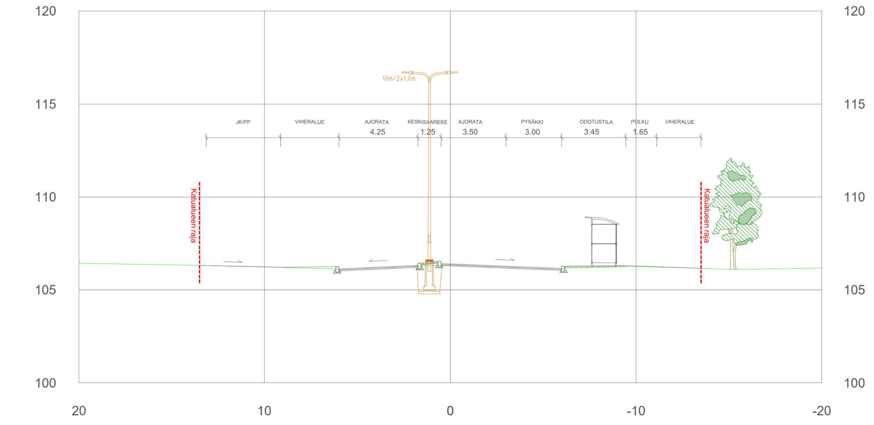
B-B PL350 / 1:100
